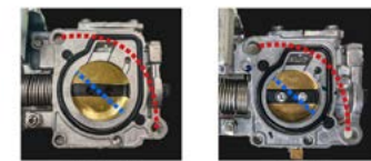
套件組 孔距 73mm 口徑 32mm、34mm 原廠 65mm 29mm
