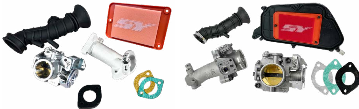
JET-S(六期)/JET-SR – 進氣套件組 適用 :FNX-125(六期) 、FIDDLE (馬桶會干涉·需自行修改)
